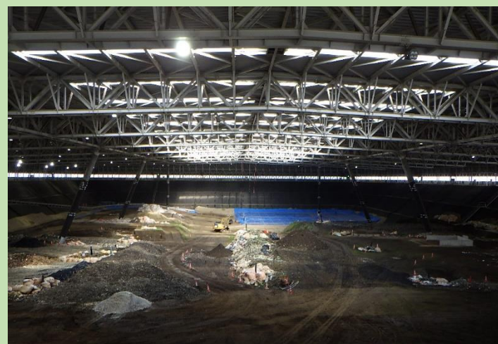
「エコアくまもと」 覆蓋施設の埋立状況
